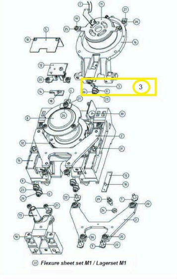
14. Weighing cell / Wägezelle
